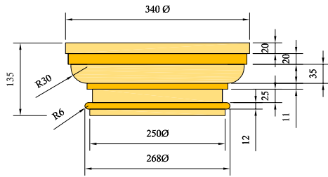
Capital
