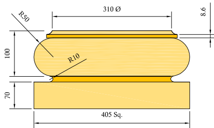
Plinth
