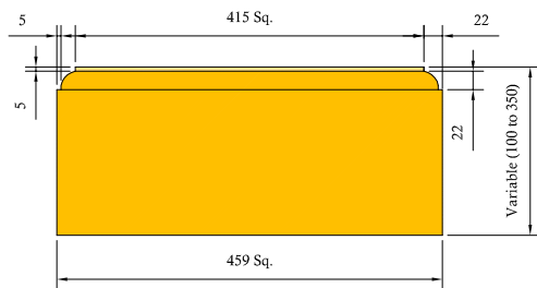
Plinth
